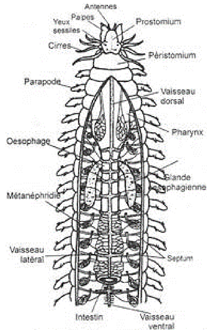
Anatomie interne polychète errante (vue dorsale)
