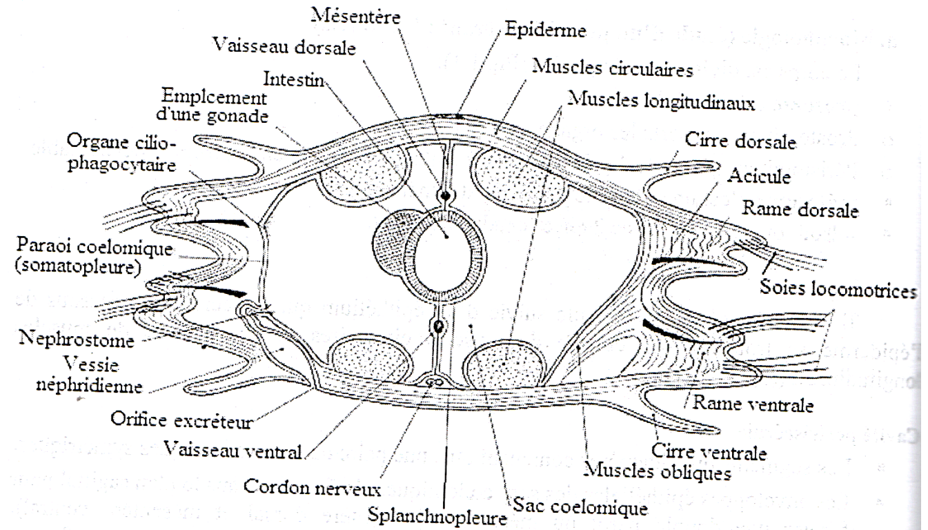
Figure 1.2. Coupe transversale au niveau d'un métamère Polychète (Néréis).
