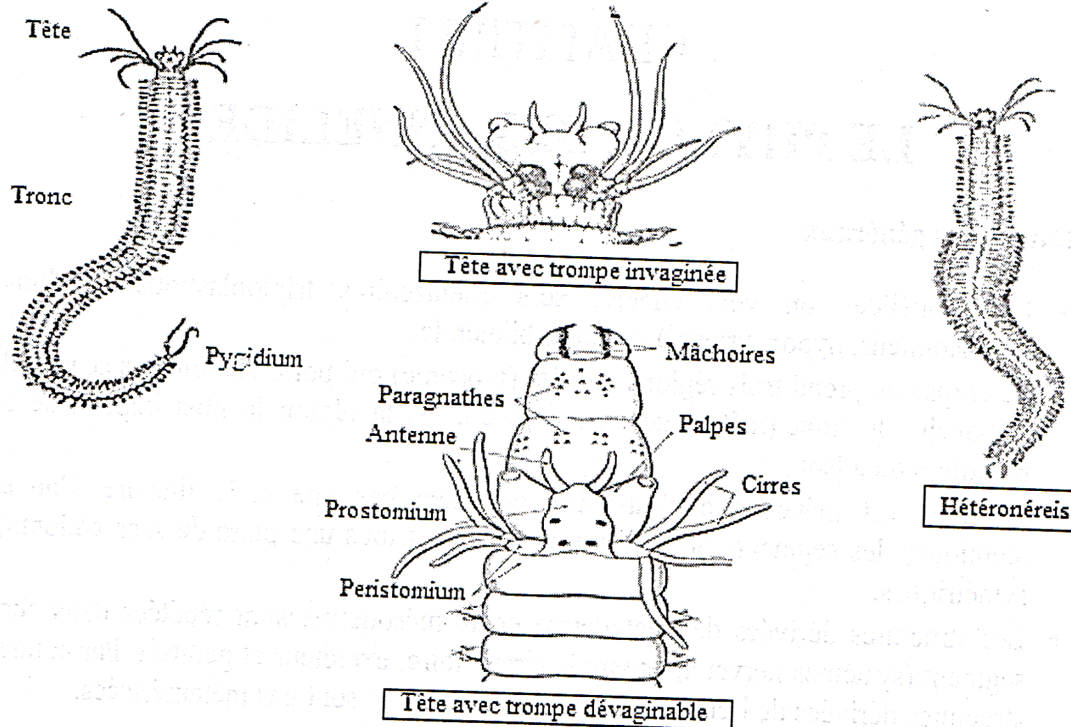
Figure 1.1. Morphologie d'un Polychète (Néréis).
