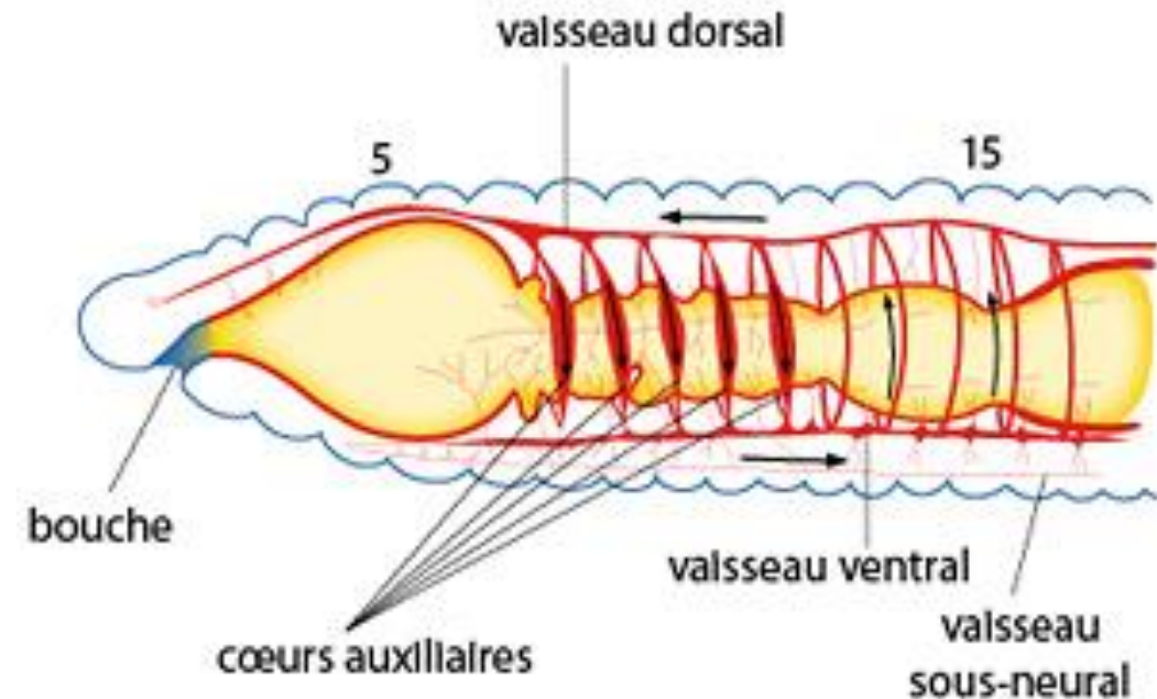
Système circulatoire d'un annélide
