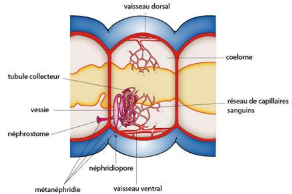
Système excréteur d'un annélide
