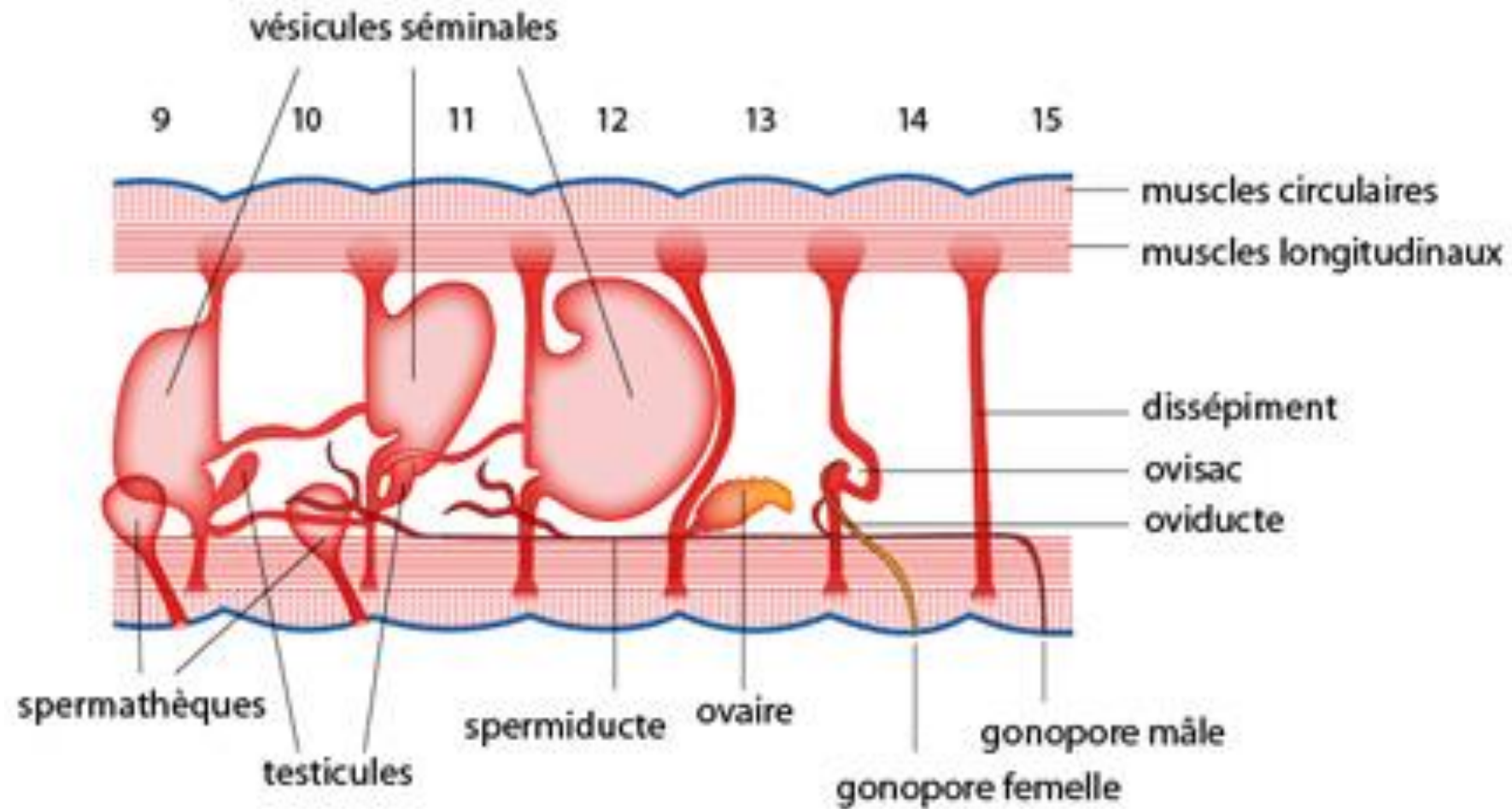
Système reproducteur d'un annélide
