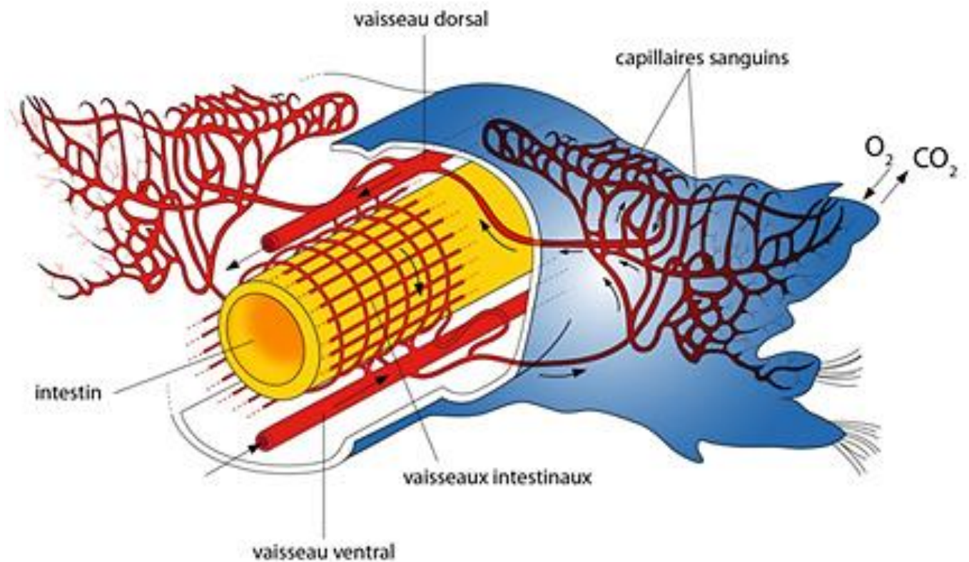
Le système circulatoire clos d'un polychète : respiration et circulation au niveau des parapodes
