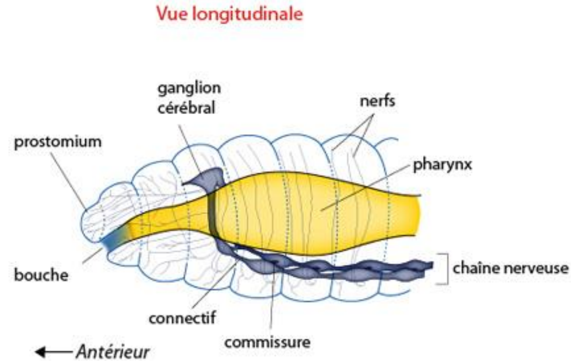
Système nerveux d'un annélide
