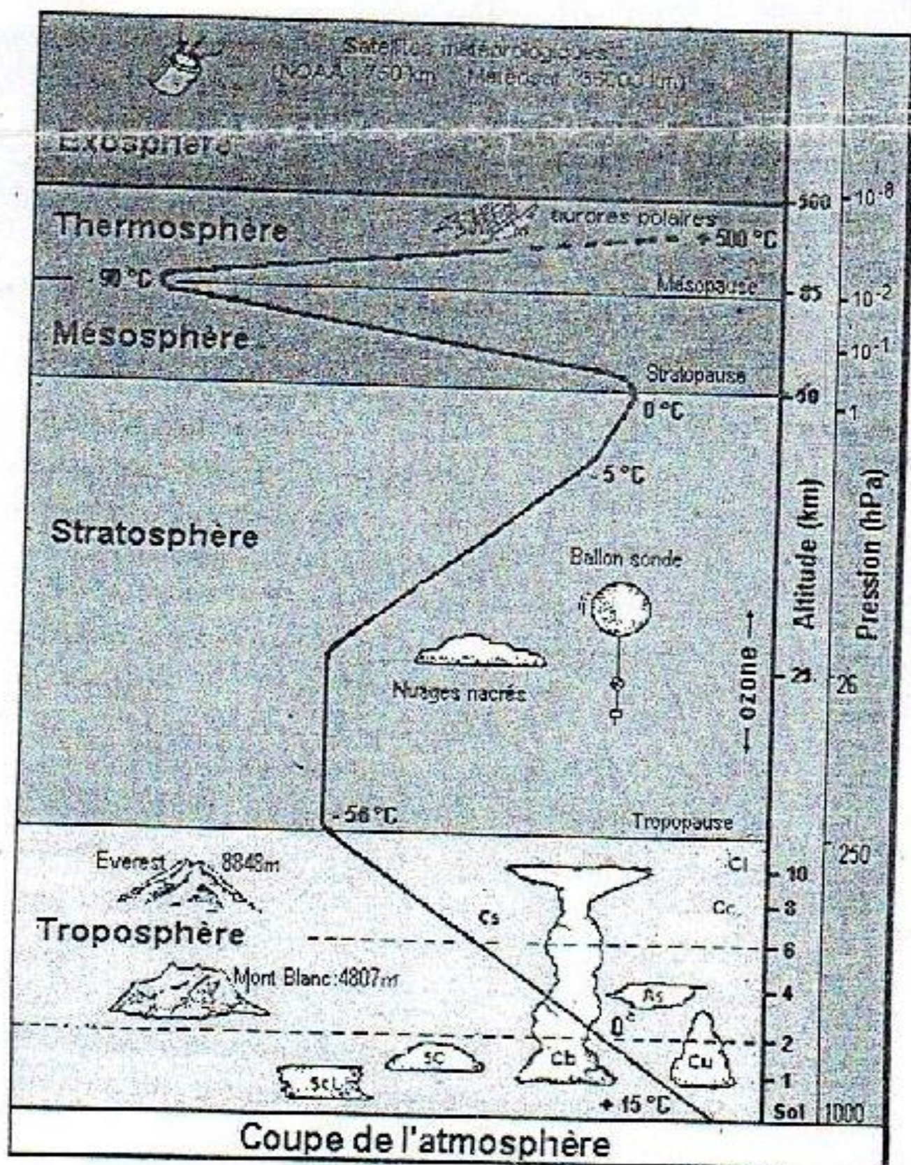
Figure 4: Différentes couches de l'atmosphère suivant l'altitude.
